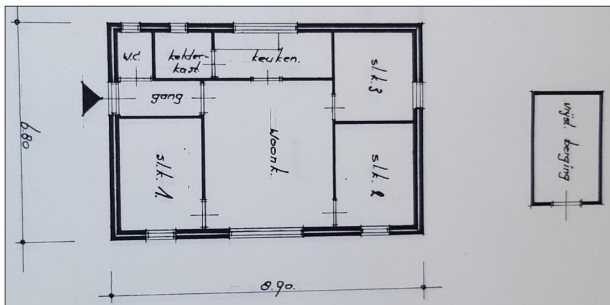
Foto 2: Plattegrond van begane grond van woningwetwoning uit 1947. Te zien zijn hal, woonkamer, keuken, drie slaapkamers, wc en kelderkast. Rechts in tuin vrijstaande berging. Bron: Gemeentearchief Horst.
